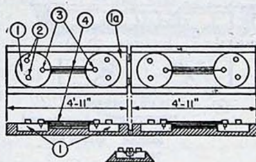
FIGURE 40.—Kammeiermine (Kammeier's mine).
