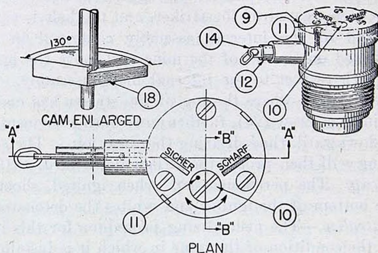
FIGURE 12.—Pressure igniter T. Mi. Z. 35.
