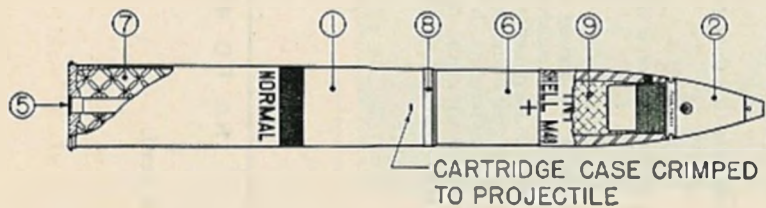
FIXED--A
