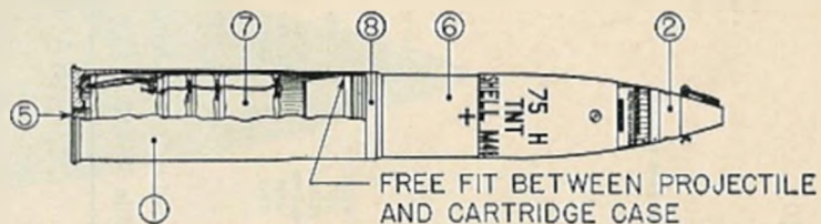
SEMIFIXED--B
