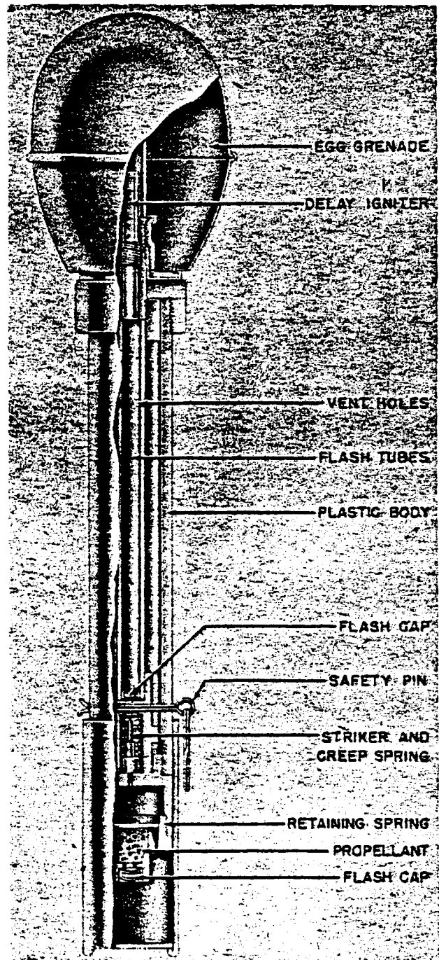
Figure 309—27-mm Pistol Grenade
