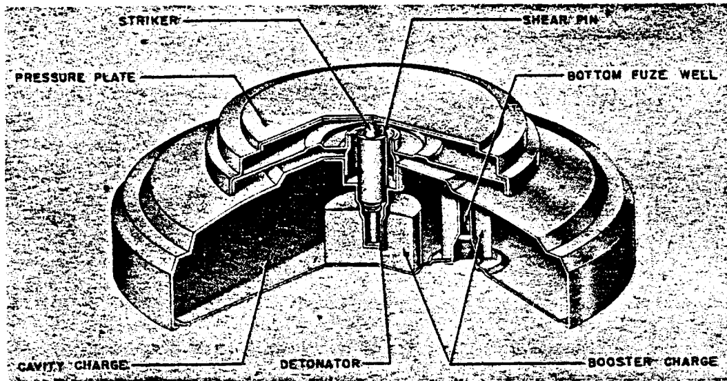
Figur 233—Tellermine 43—Antitank
