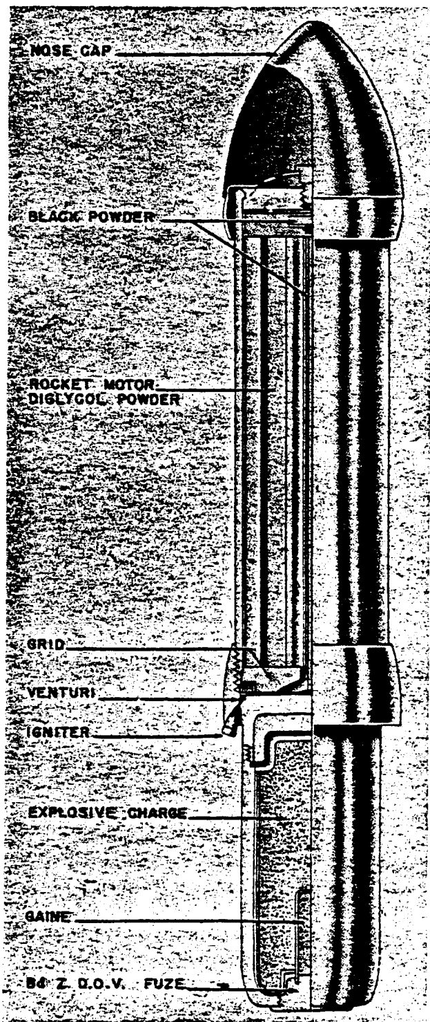
Figure 211—15-cm H. E. Rocket
