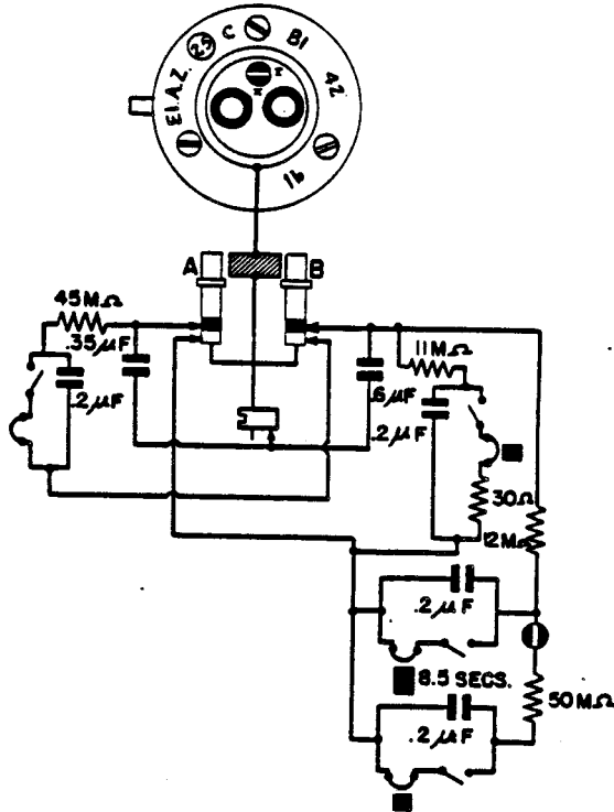
Figure 142—(25)C Electrical Impact Fuze
