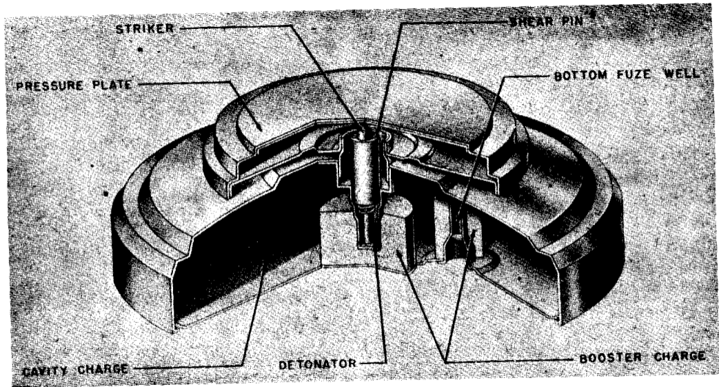
Figur 233—Tellermine 43—Antitank
