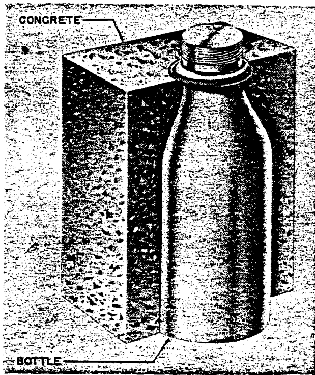
Figure 247—Eismine 42—Antipersonnel
