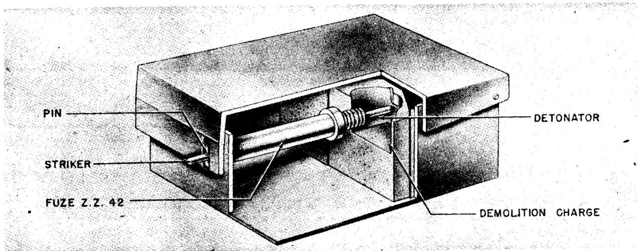
Figure 243—Schumine 42—Antipersonnel
