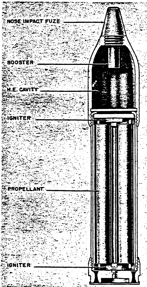
Figure 221—8.6-cm R. Spgr L/5.5 Rocket
