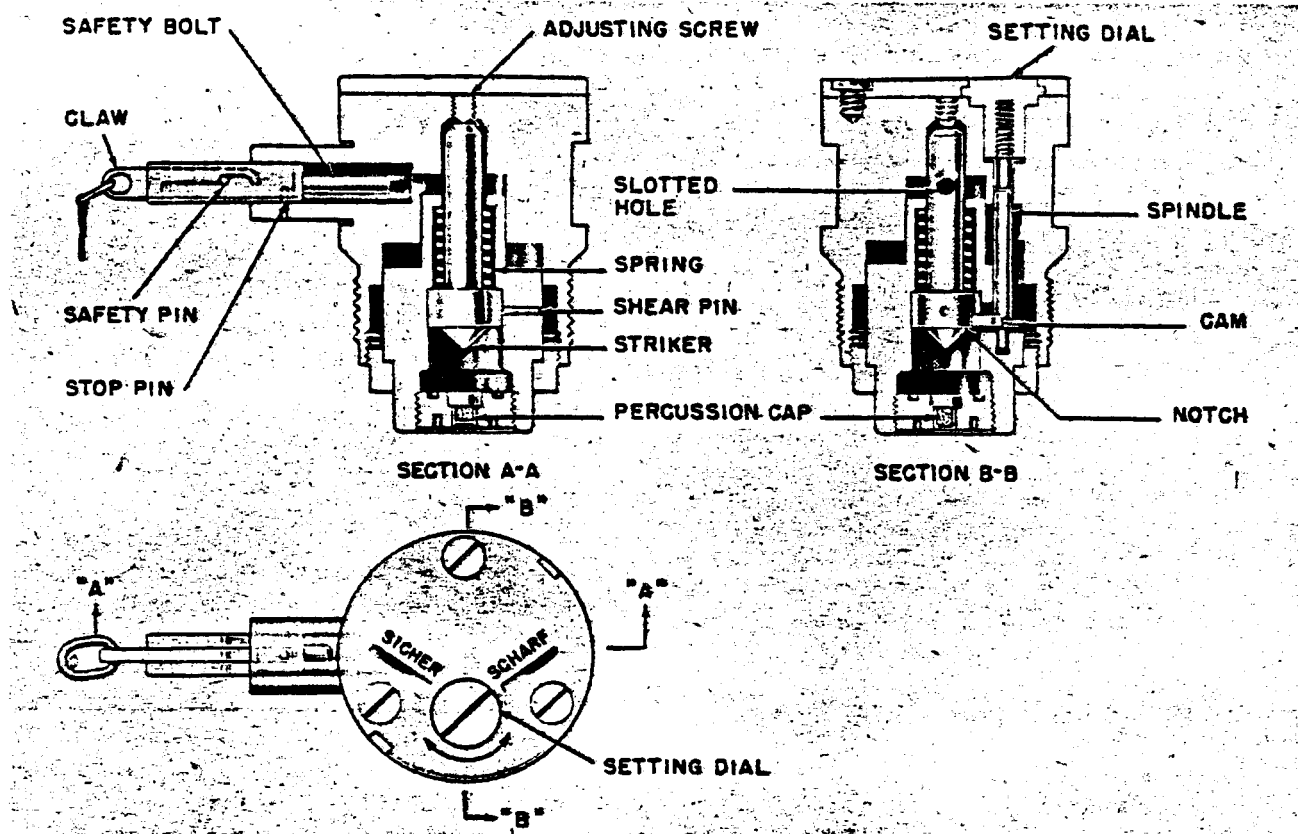
Figure 269—T. Mi. Z. 35 Pressure Igniter
