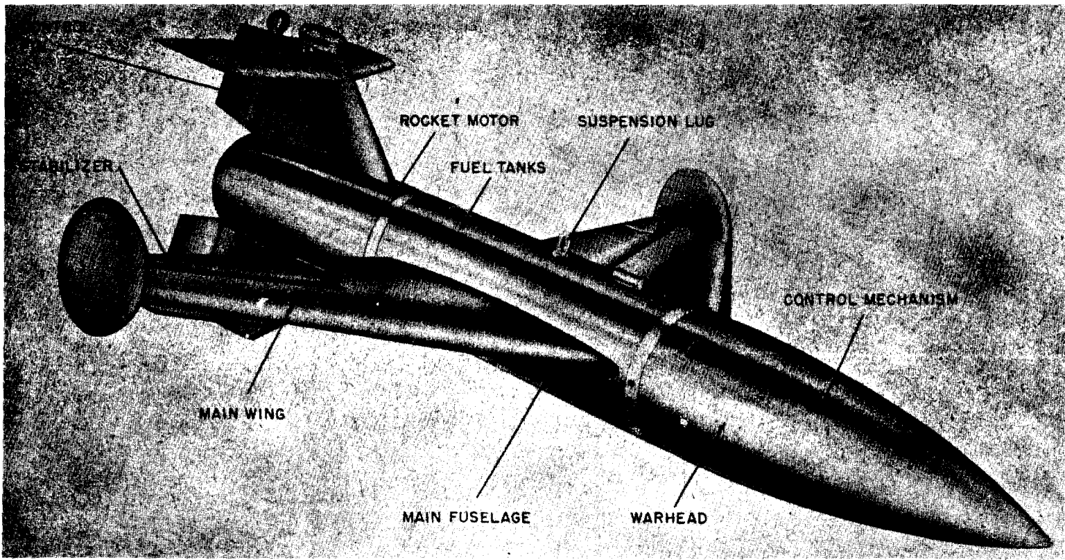
Figure 200—Feuerlilie F-25; Feuerlilie F-55
