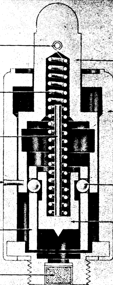
Figure 271—T. Mi. Z. 43 Pressure Igniter
