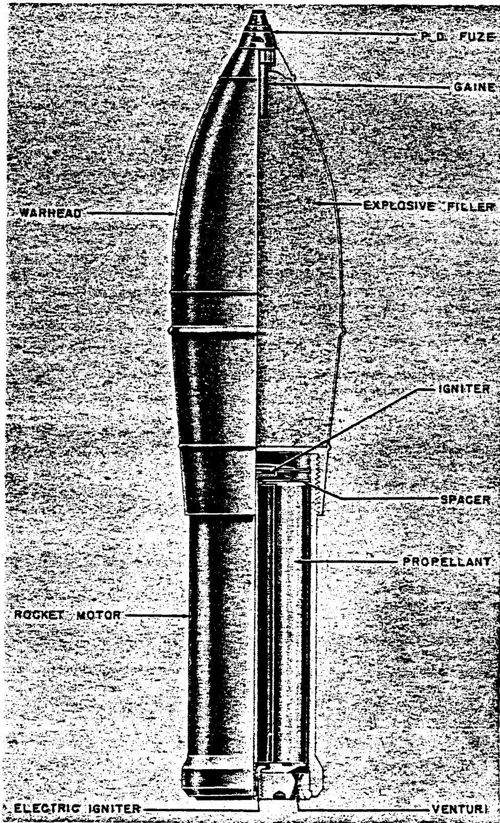
Figure 217—30-cm H. E. Rocket
