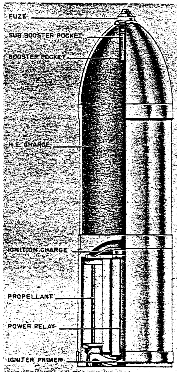
Figure 219—38-cm H. E. Rocket
