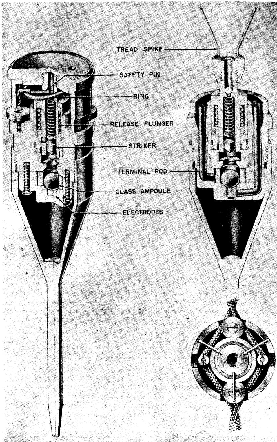
Figure 268—E. S. Mi. Z. 40 Pressure Igniter (Electric)
