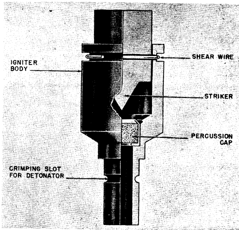
Figure 274—Fi. Es. Mi. Z. Pressure Igniter
