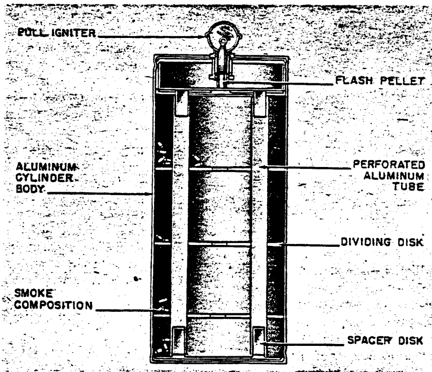
Figure 84—Smoke Signal Flare A. R. D. R.
