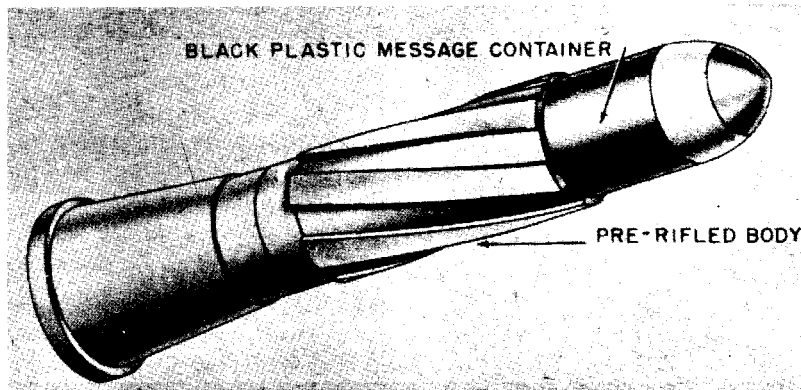
Figure 314—27-mm Message Pistol Grenade
