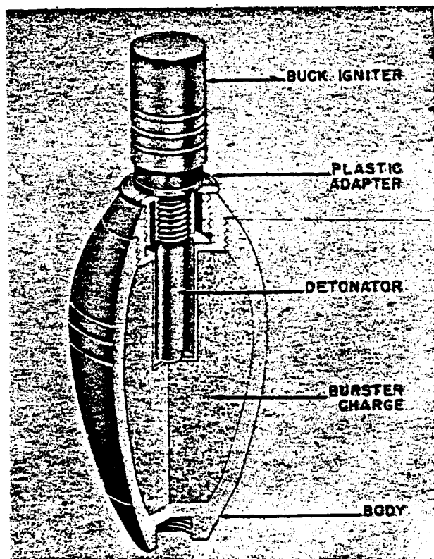
Figure 244—Behelfsmine W-1—Antipersonnel
