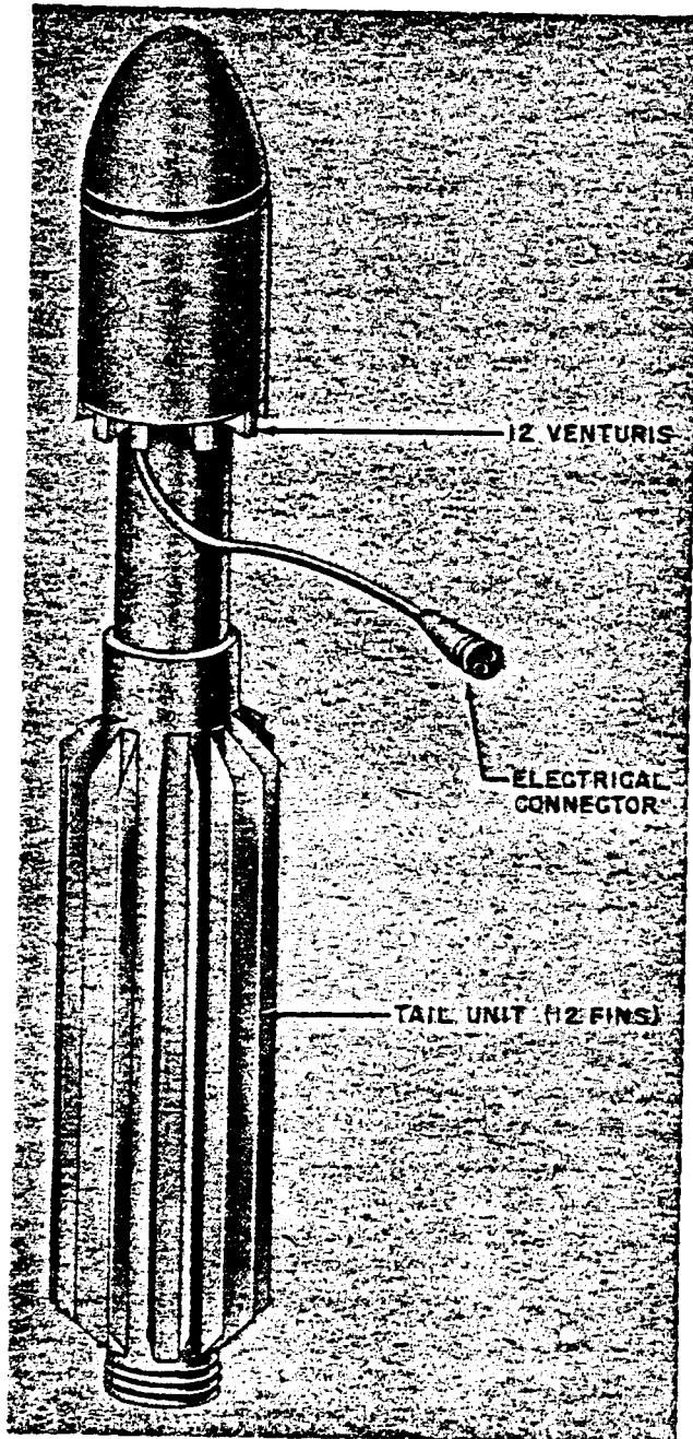
Figure 214—20-cm Antiaircraft Rocket
