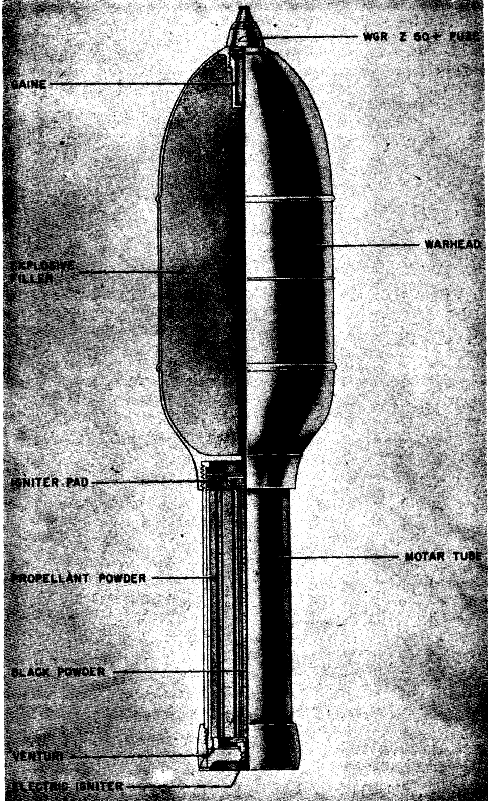
Figure 216—28-cm H. E. Rocket
