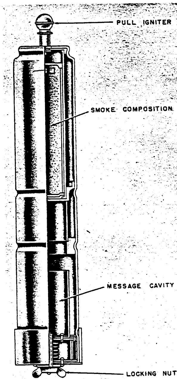
Figure 118—Message Tube (land)
