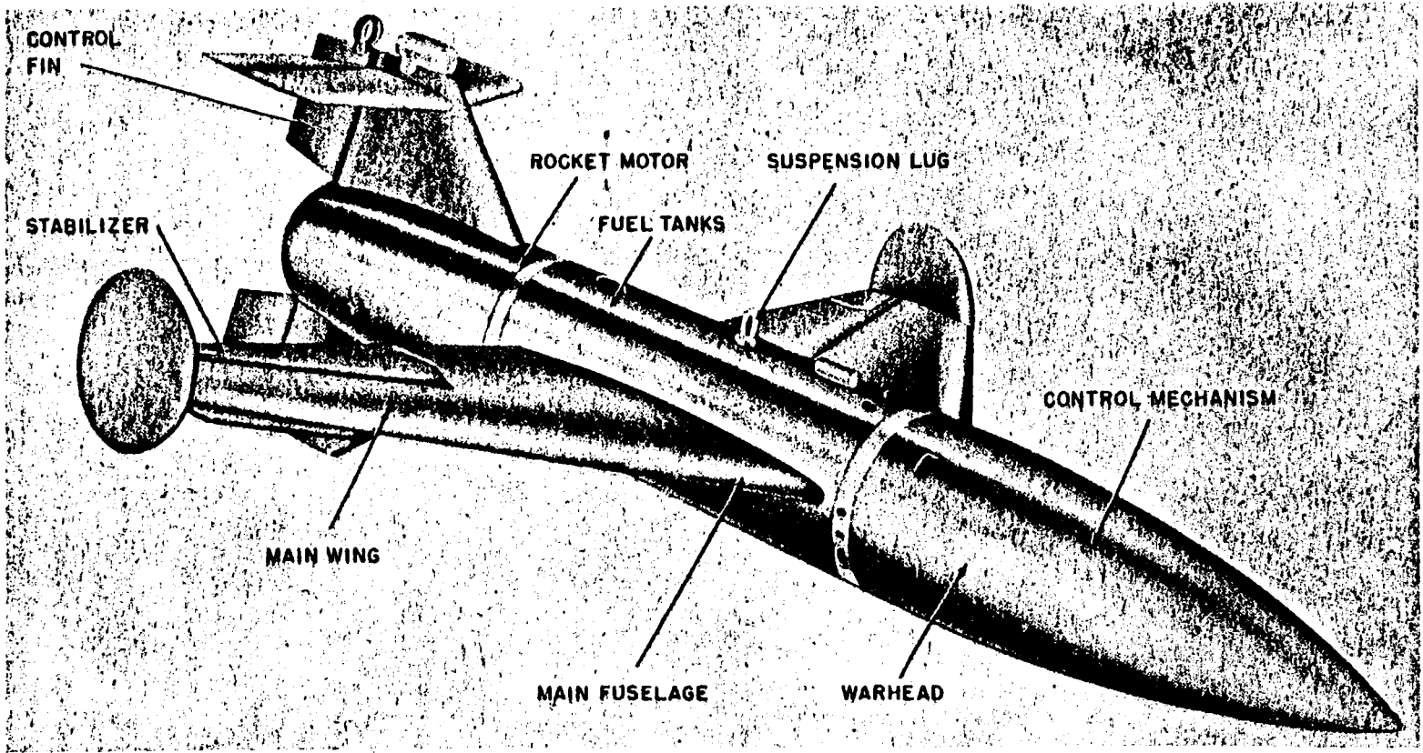
Figure 200—Feuerllille F-25; Feuerllille F-55
