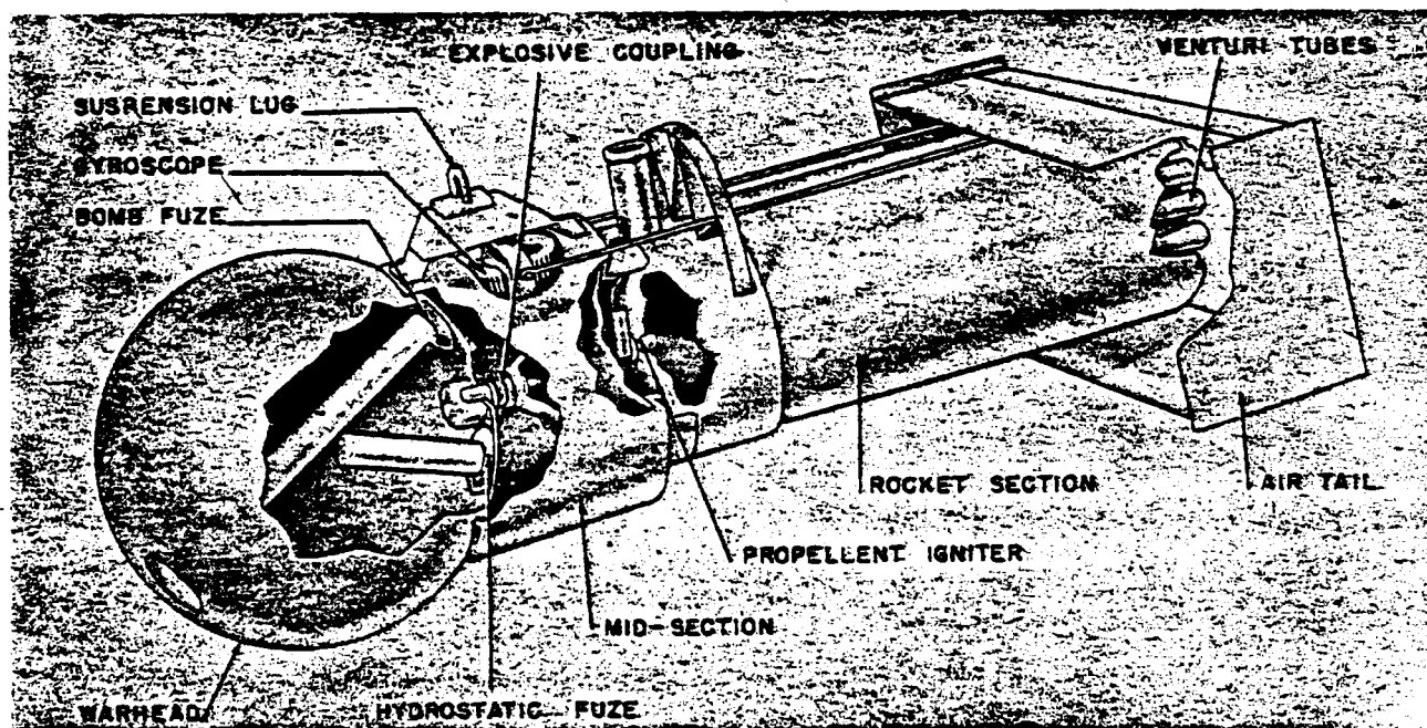
Figure 19—SB 400 Skip Bomb (Kugel K-Kurt Apparatus)
