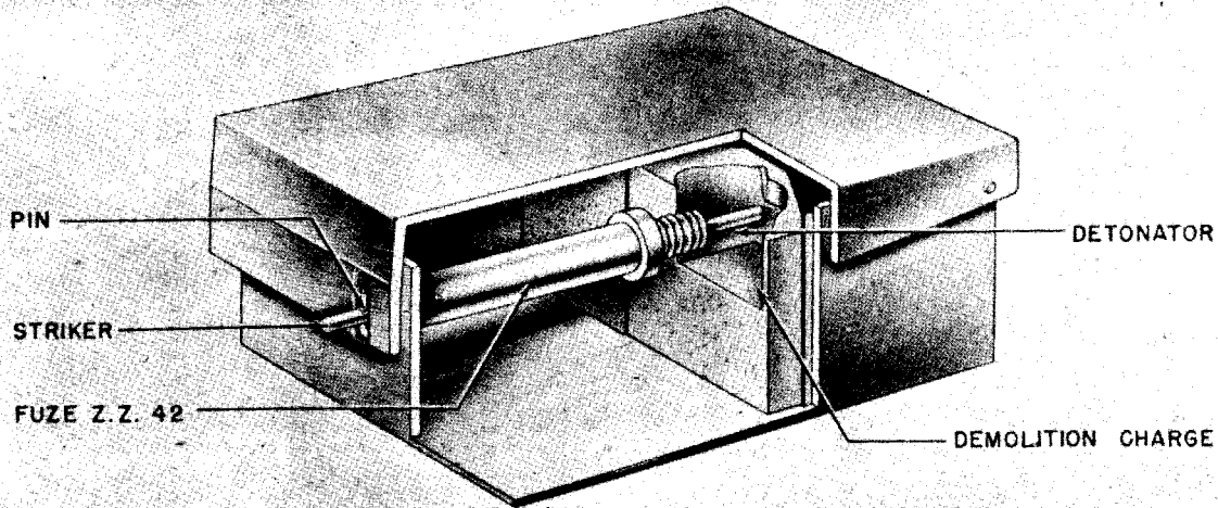
Figure 243—Schumine 42—Antipersonnel
