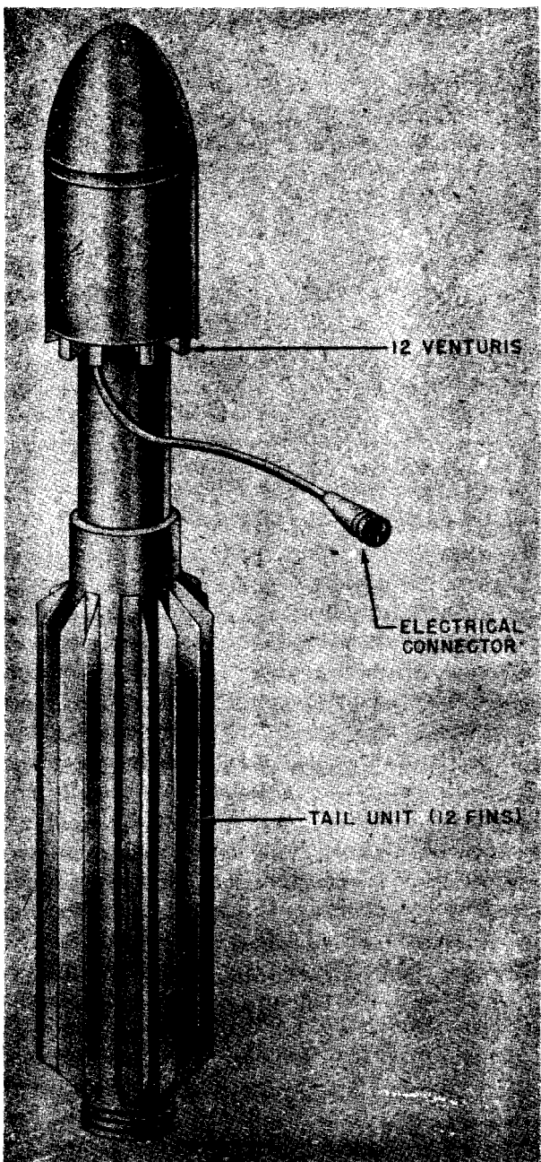
Figure 214—20-cm Antiaircraft Rocket
