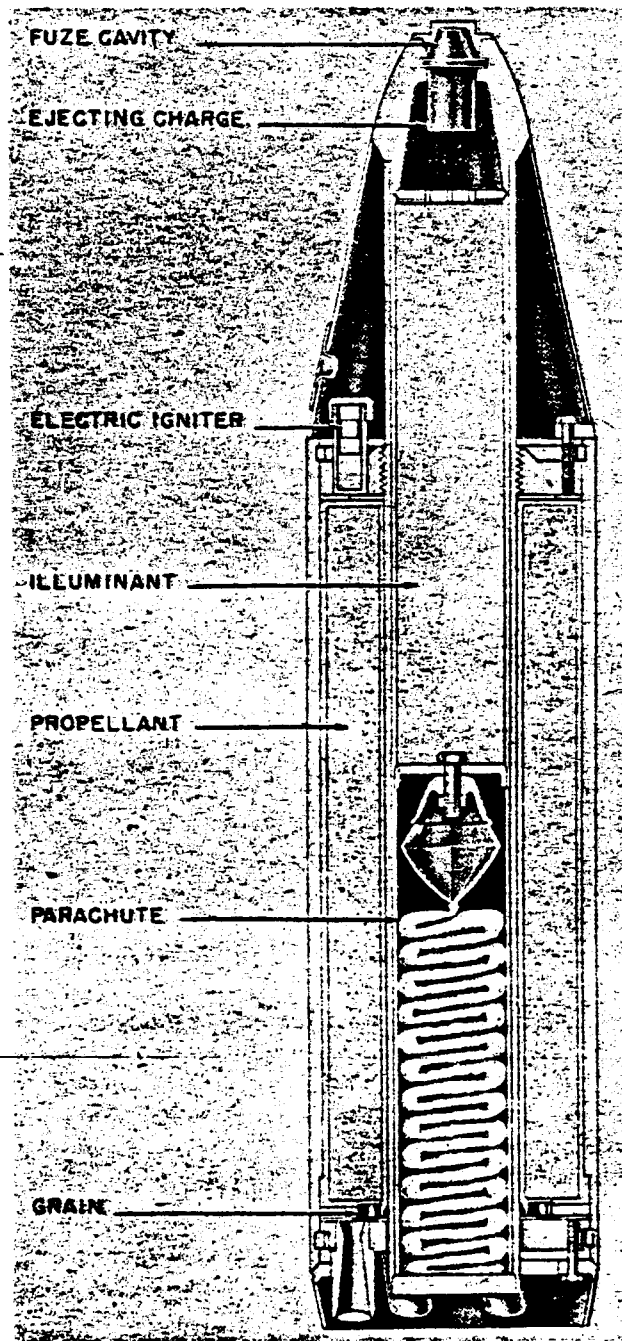
Figure 223—21-cm R-Lg Rocket
