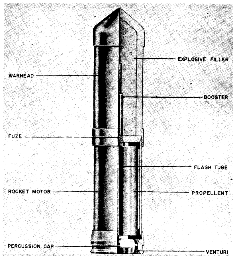
Figure 207—8.6-cm H. E. Rocket (Naval)
