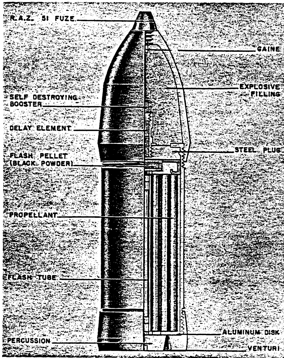
Figure 205—7.3-cm R. Sprgr Rocket
