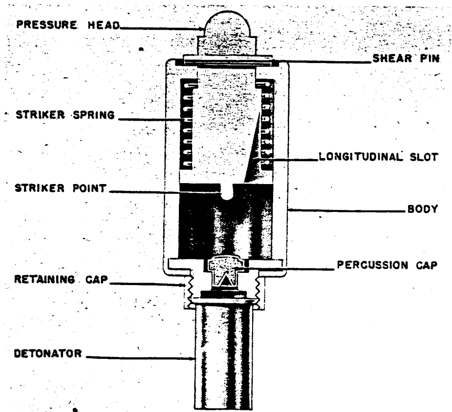
Figure 270—T. Mi. Z. 42 Pressure Igniter
