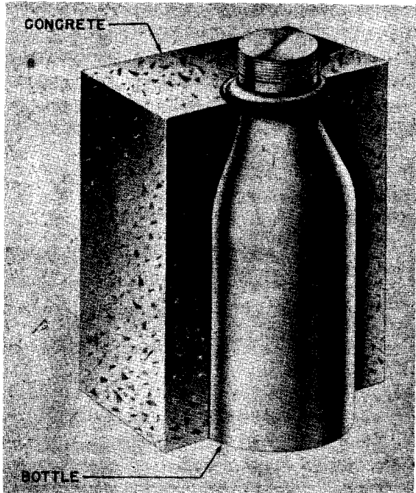
Figure 247—Eismine 42—Antipersonnel
